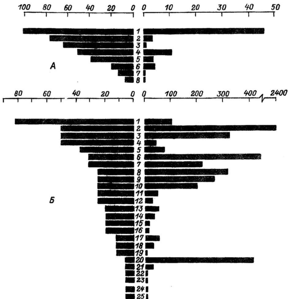
Рис. 1. Зараженность куланов отдельными видами стронгилид.
