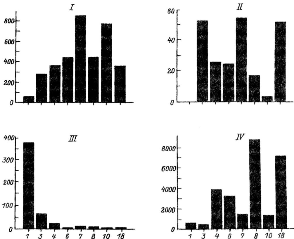
Рис. 2. Зависимость интенсивности заражения от возраста хозяина.
